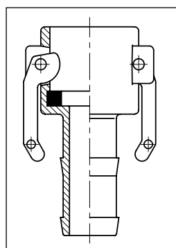
Camlock, hun slangestuss
