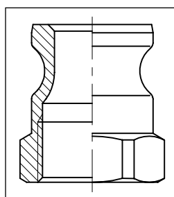
Camlock, han innv. gjenge
